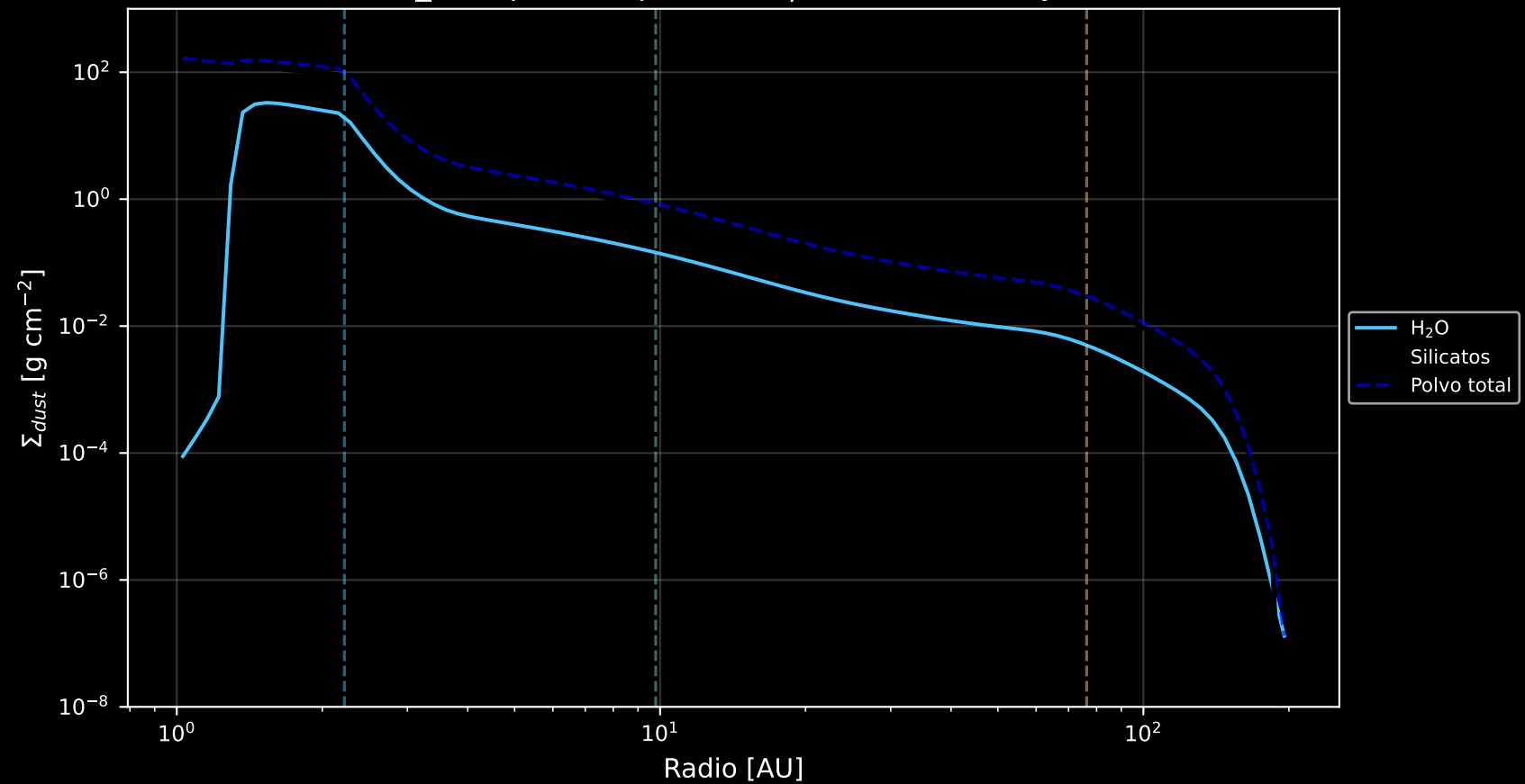
\Sigma_{dust} por componente | t = 1.00e+05 yr
